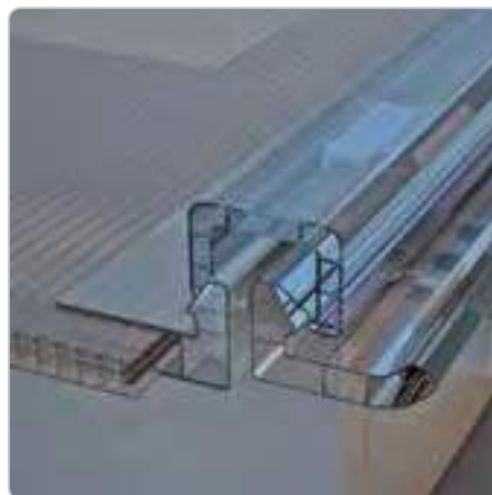
PROFIL SFÂRȘIT Insertie specială "profil sfârșit" pentru finalizarea acoperișului.
